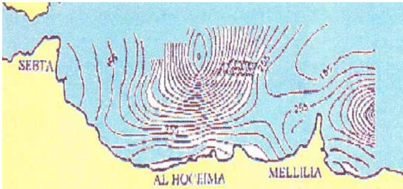
Figure 10 : Distribution du biovolume du plancton (ml/m 2 ) en mer Méditerranée marocaine (juillet 1993) (INRH 2002).
