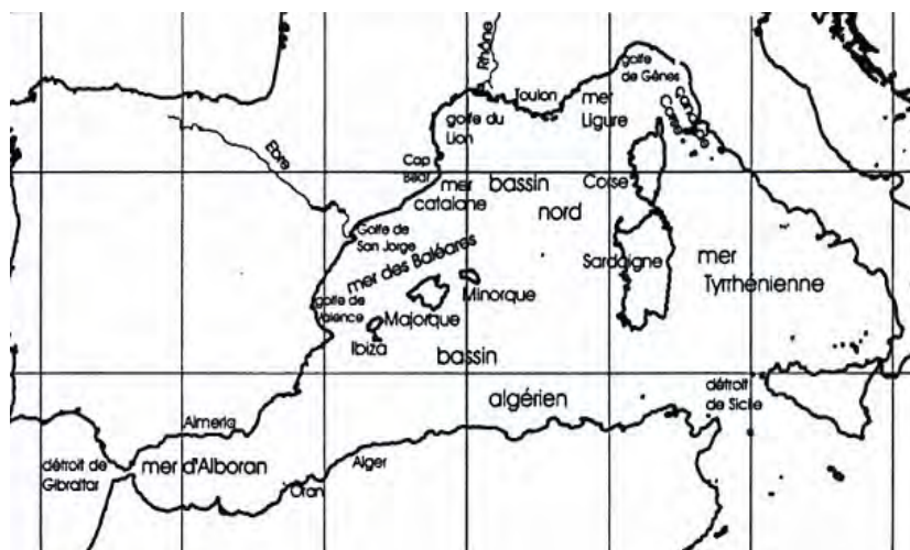
Figure 6 : Répartition des principaux bassins représentant la Méditerranée Occidentale.
