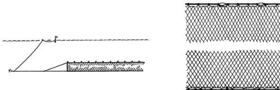
Slika 12. Jednostruke mreže stajačice
